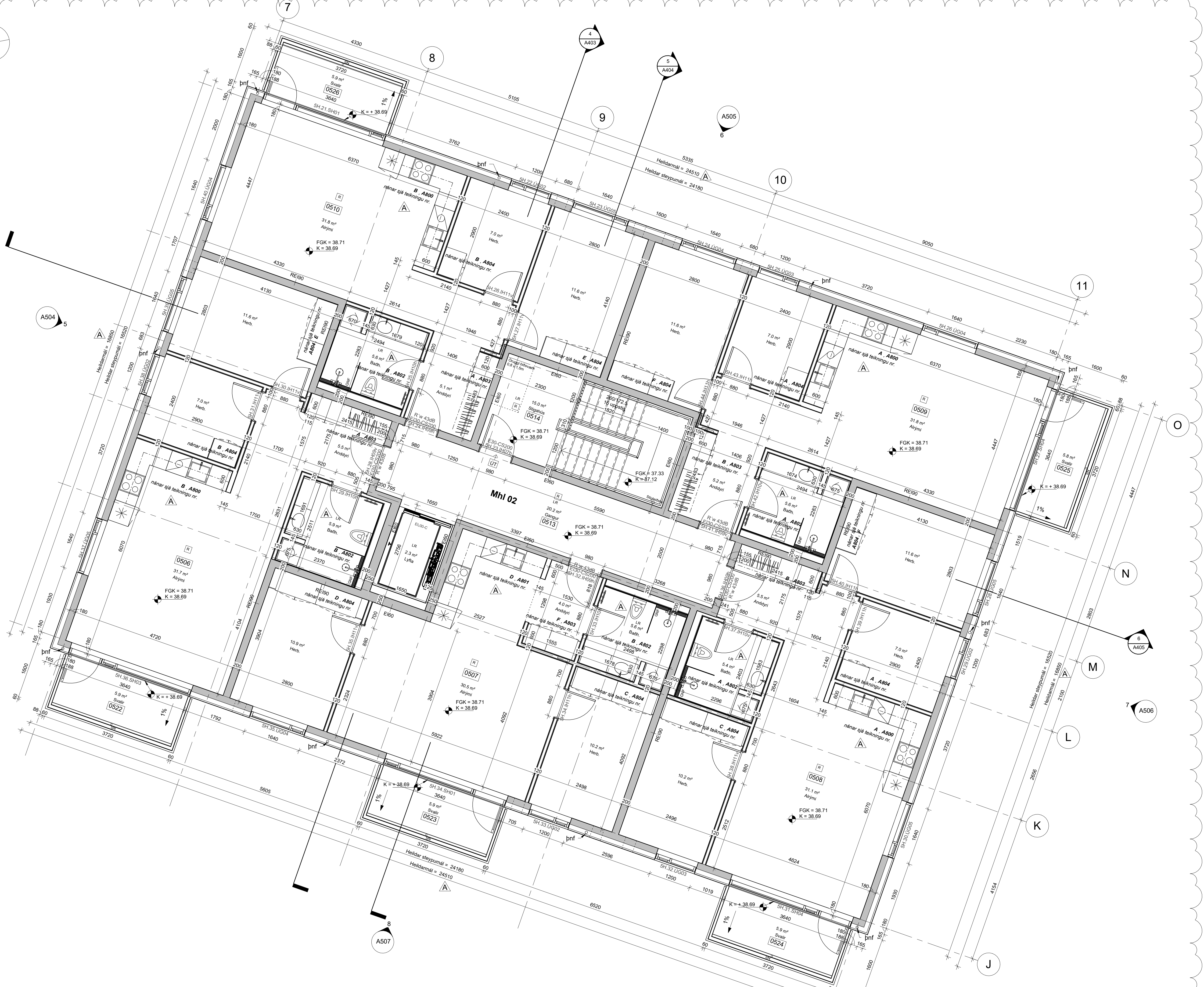
1 5. hæð - Hluti 2 - Hús nr. 29 1:50
