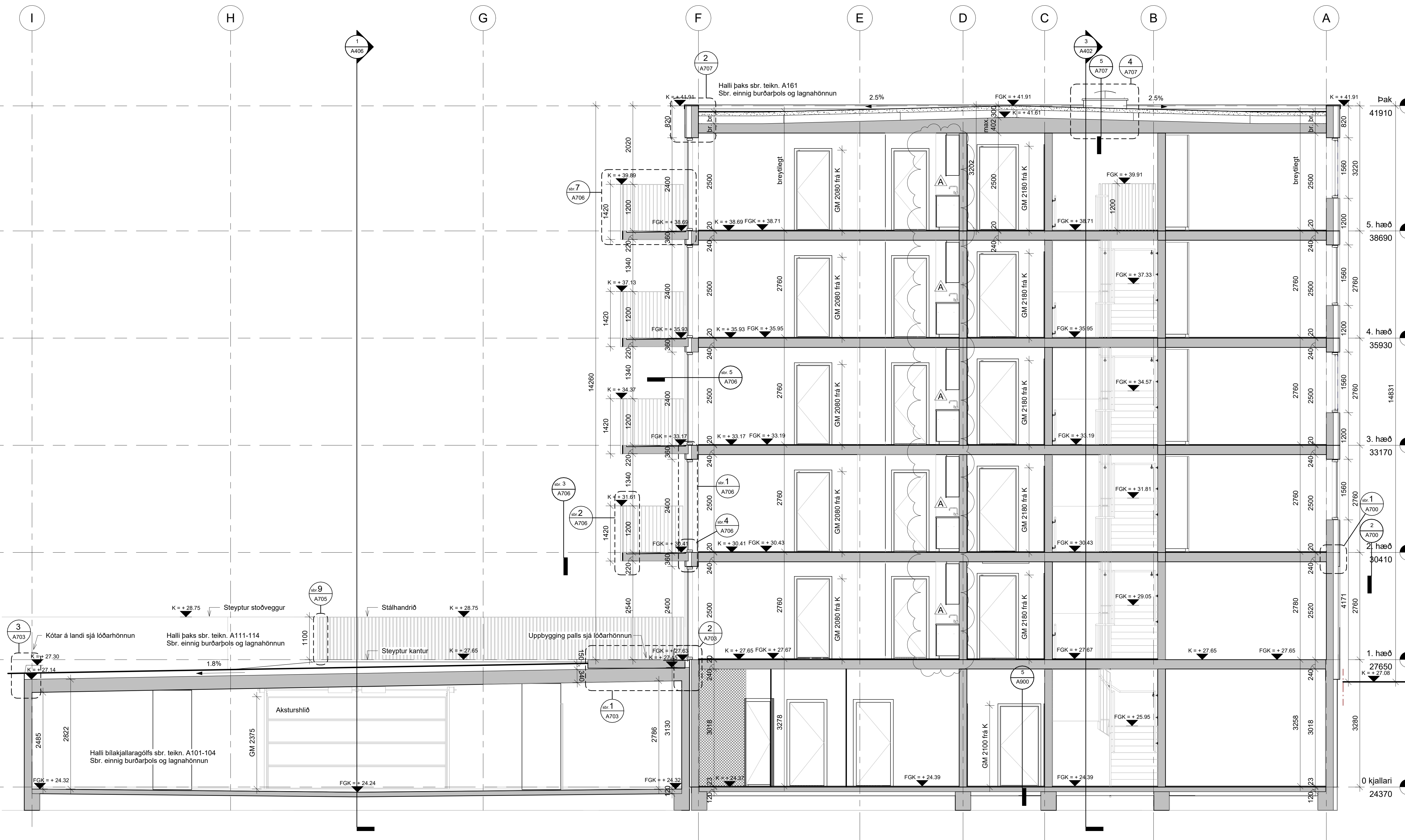
Bílakjallari Mhl 03
