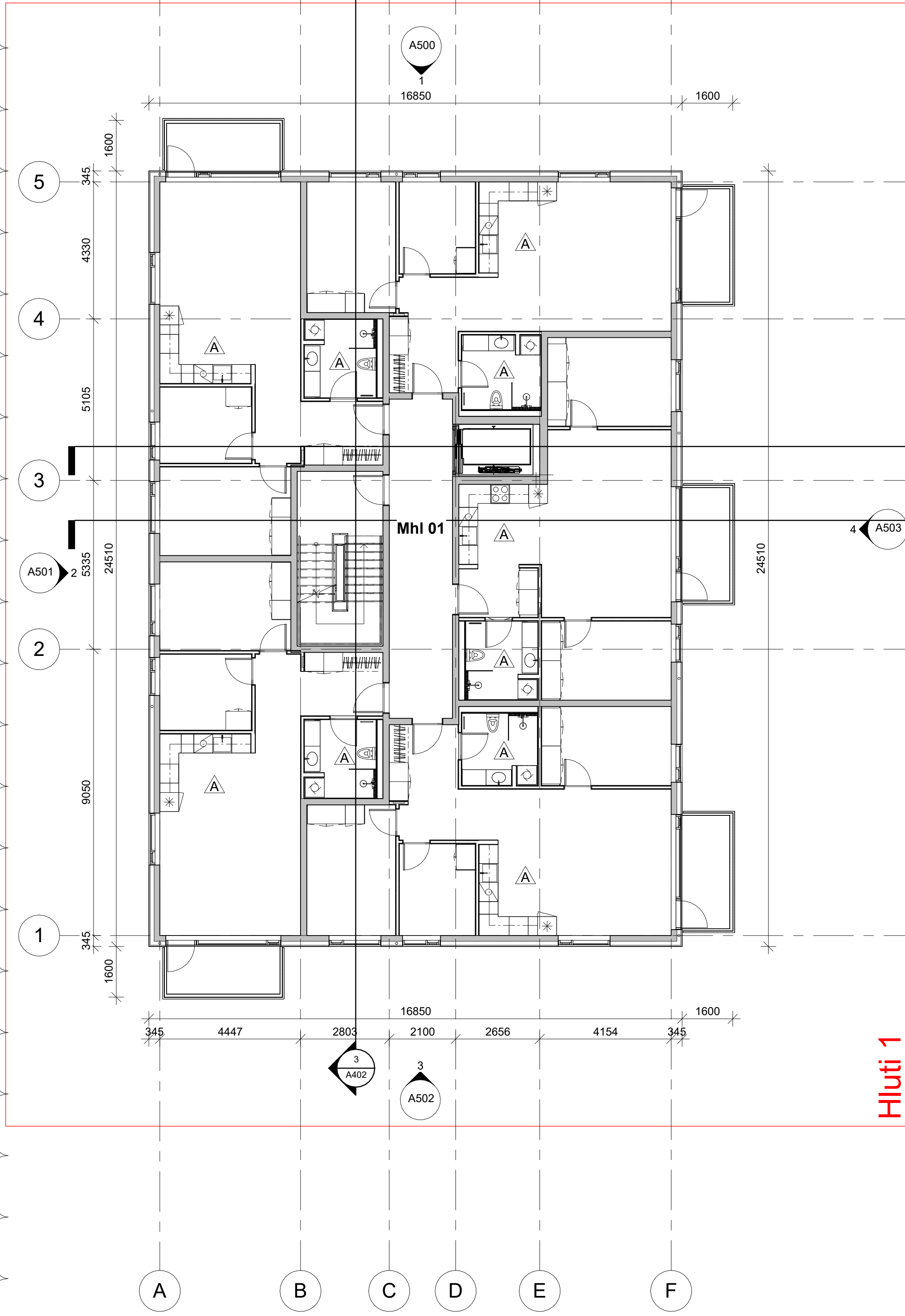
1 2. hæð, yfirlitsmynd 1 : 100
