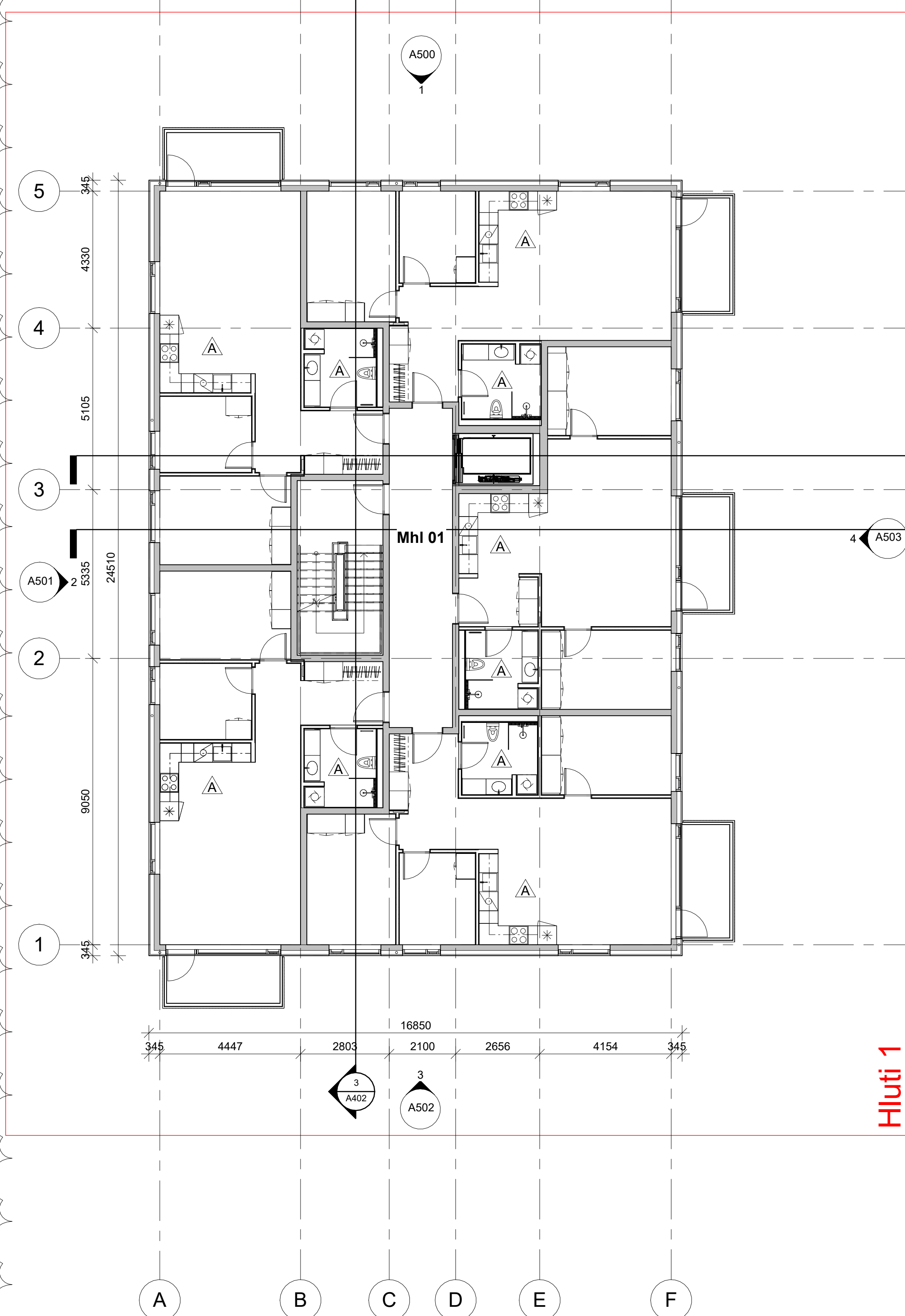
4. hæð, yfirlitsmynd 1 : 100
