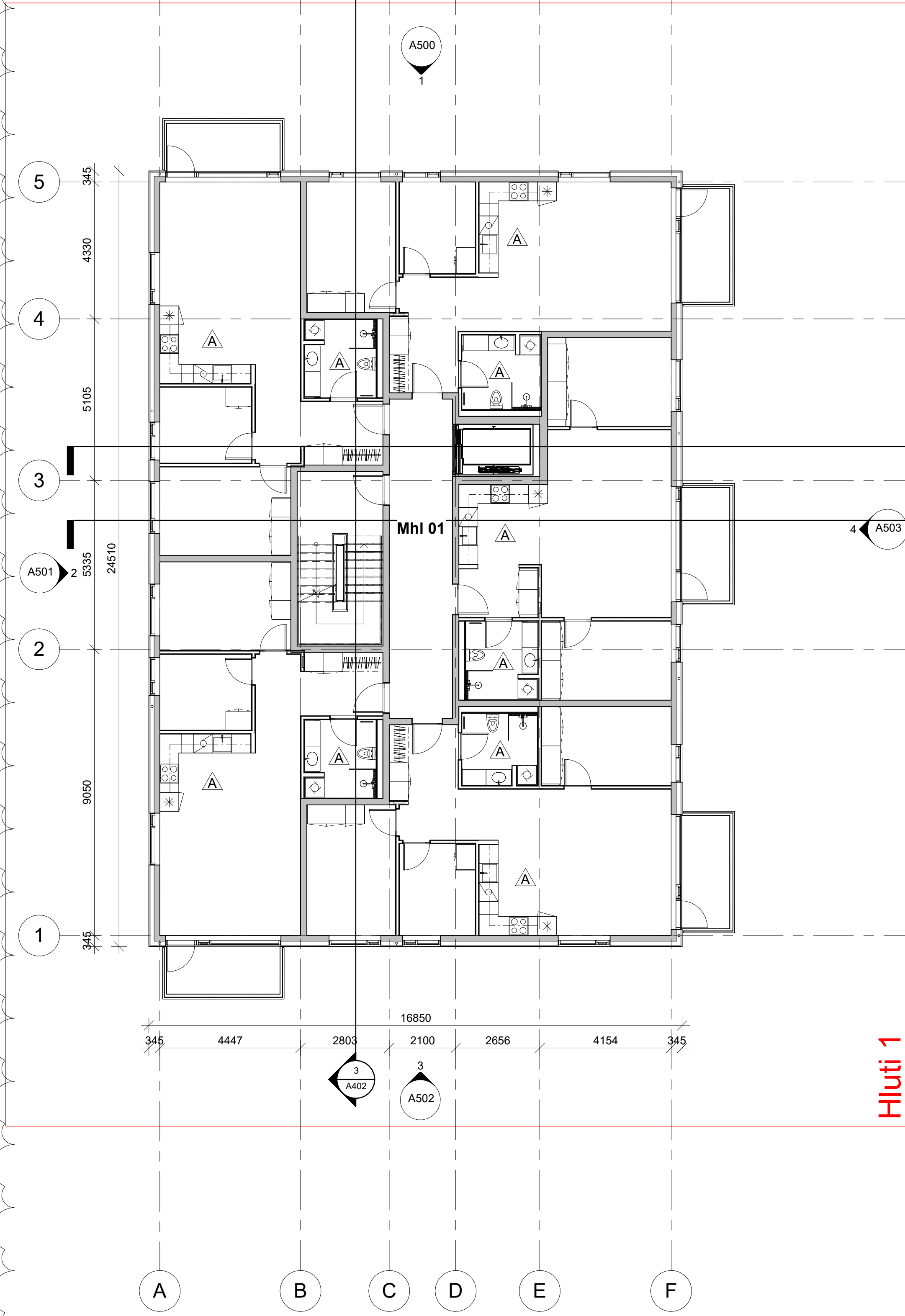
3. hæð, yfirlitsmynd 1 : 100
