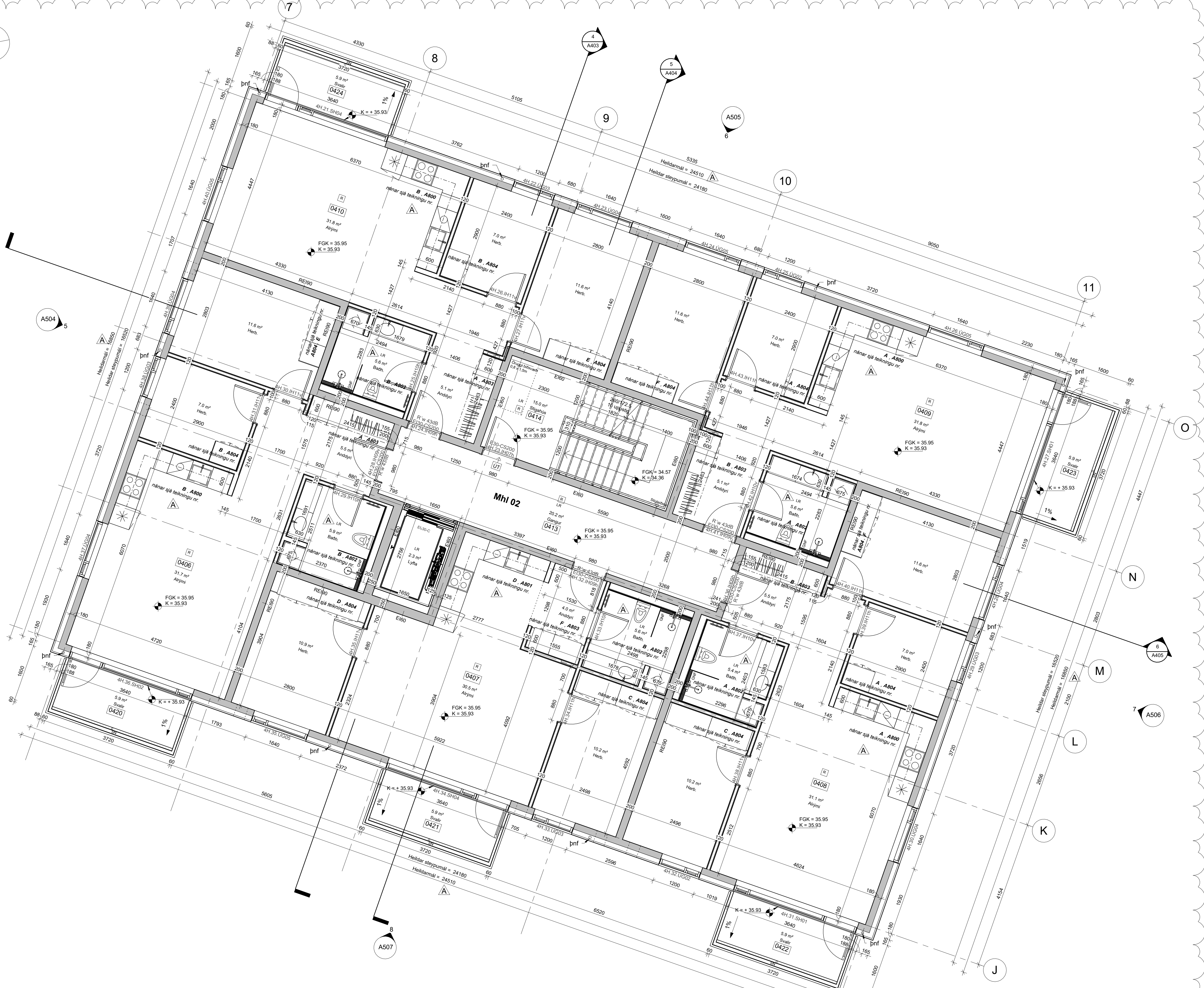
1 4. hæð - Hluti 2 - Hús nr. 29 1:50
