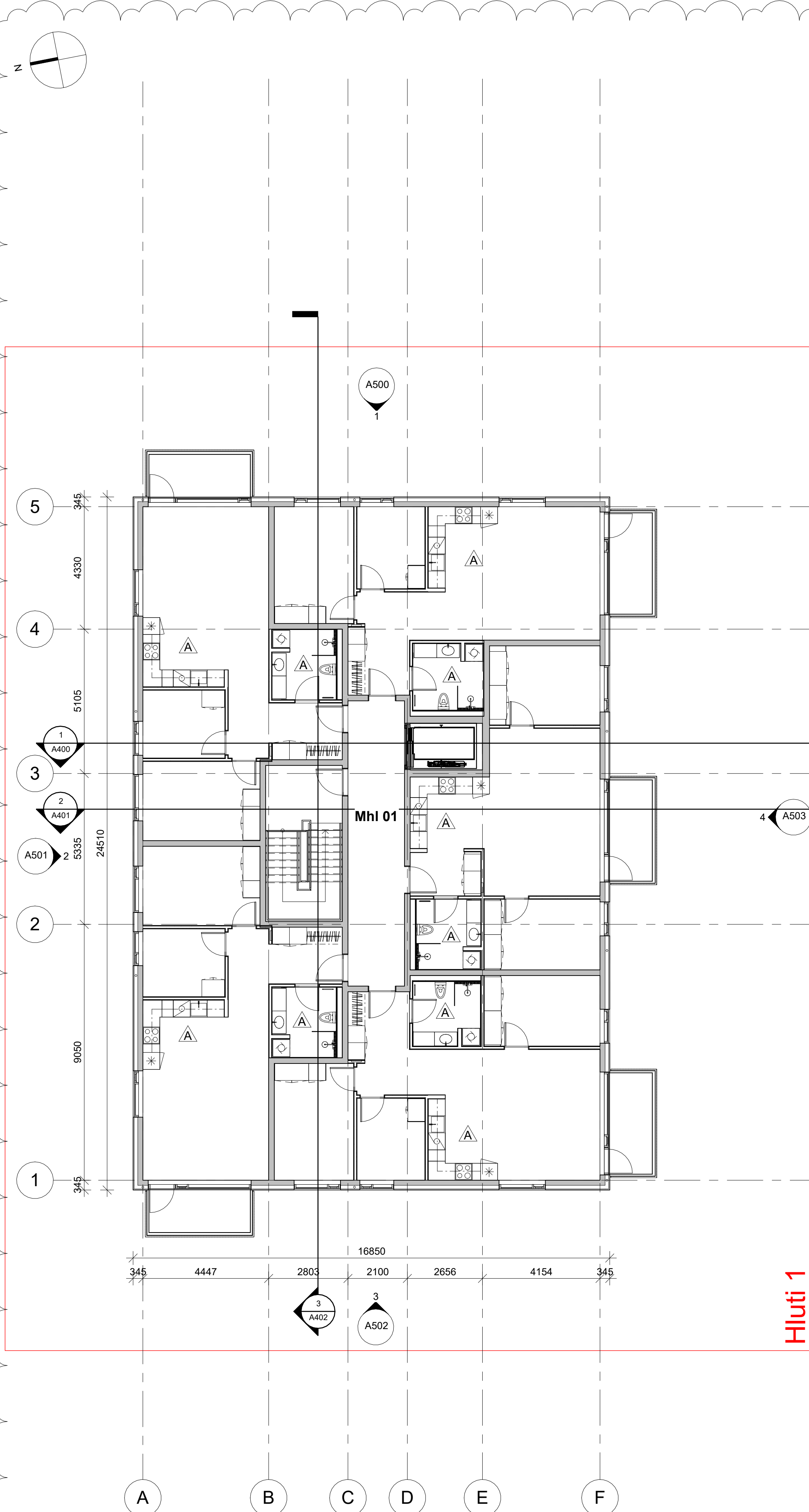
1 5. hæð, yfirlitsmynd 1 : 100
